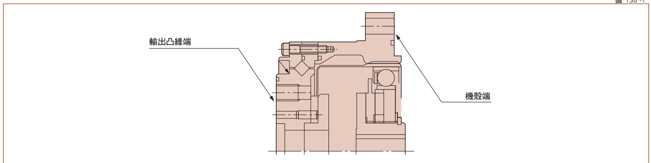
CSG 系列 輸出凸緣端的安裝及傳動轉矩
