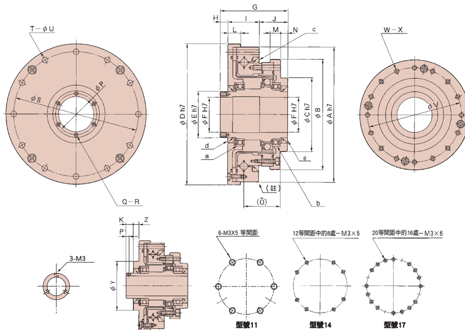
型號 14、17 的輸入部形狀
