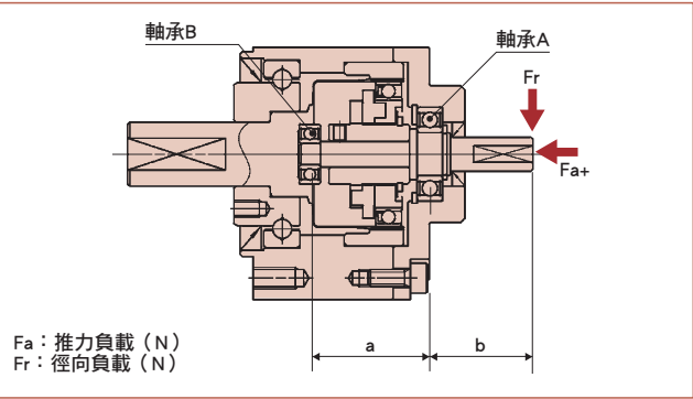
軸承支撐點
