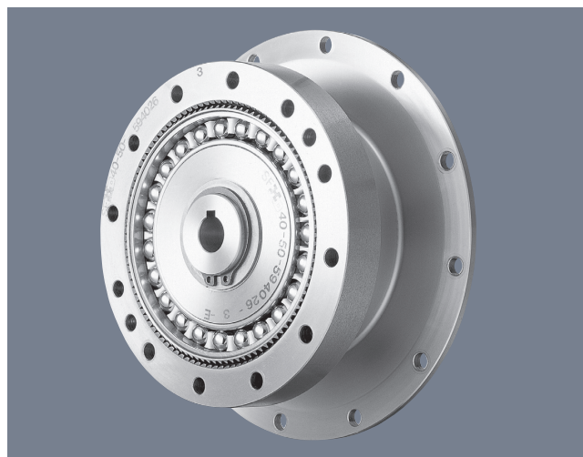
SHG / SHF 系列元件型的結構
