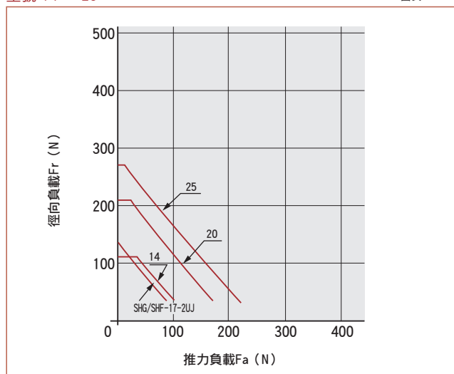
型號 14 ~ 25
