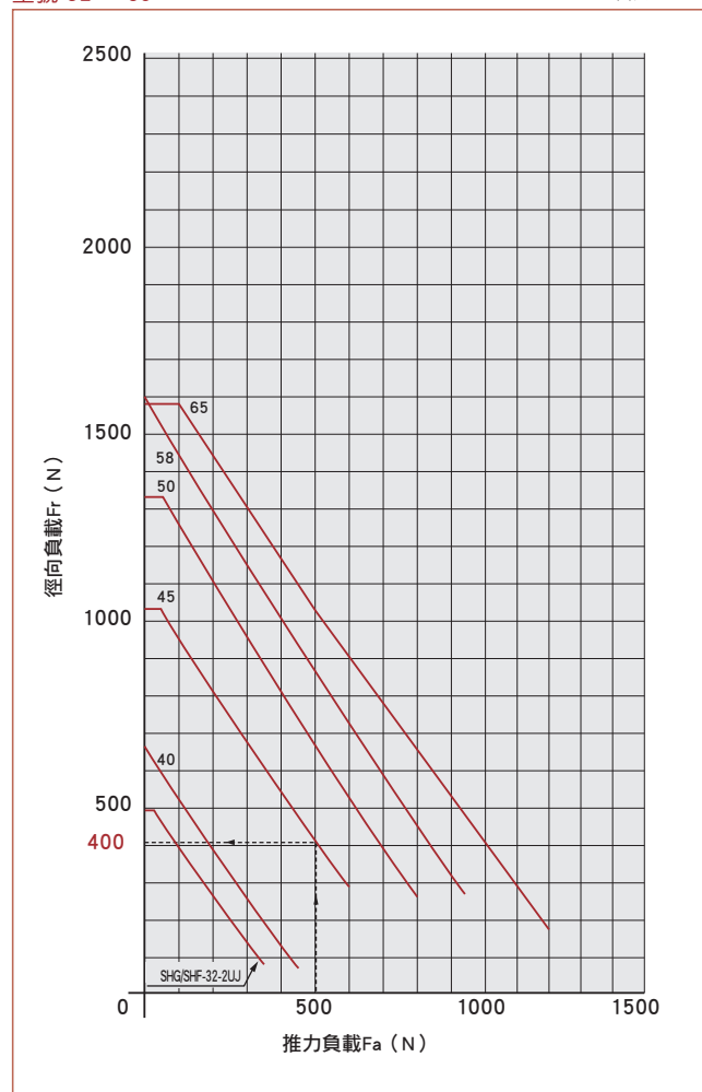
型號 32 ~ 65
