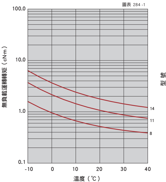
輸入轉速 500r/min
