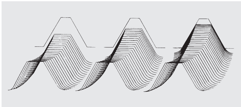
以往的齒形
