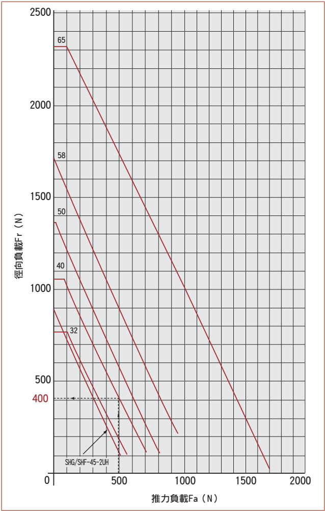
型號 32 ~ 65
