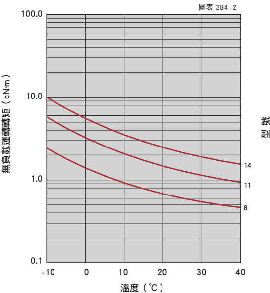
輸入轉速 1000r/min
