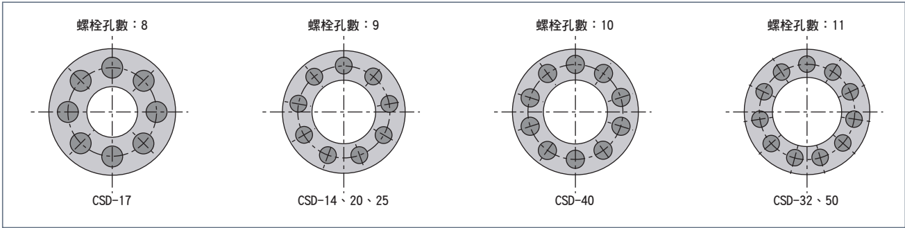
螺栓孔數及孔位置
