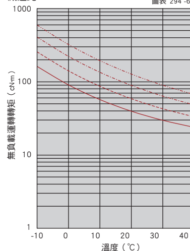
型號：32 減速比：100
