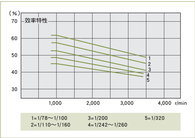
效率
