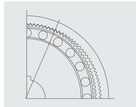
齒嚙合區域
