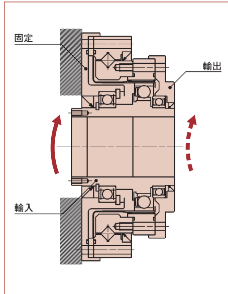
中空型 (2UH)
